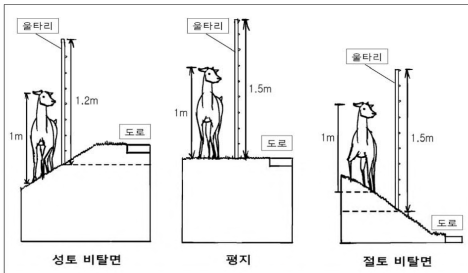
그림 3-5. 지형에 따른 울타리 높이
